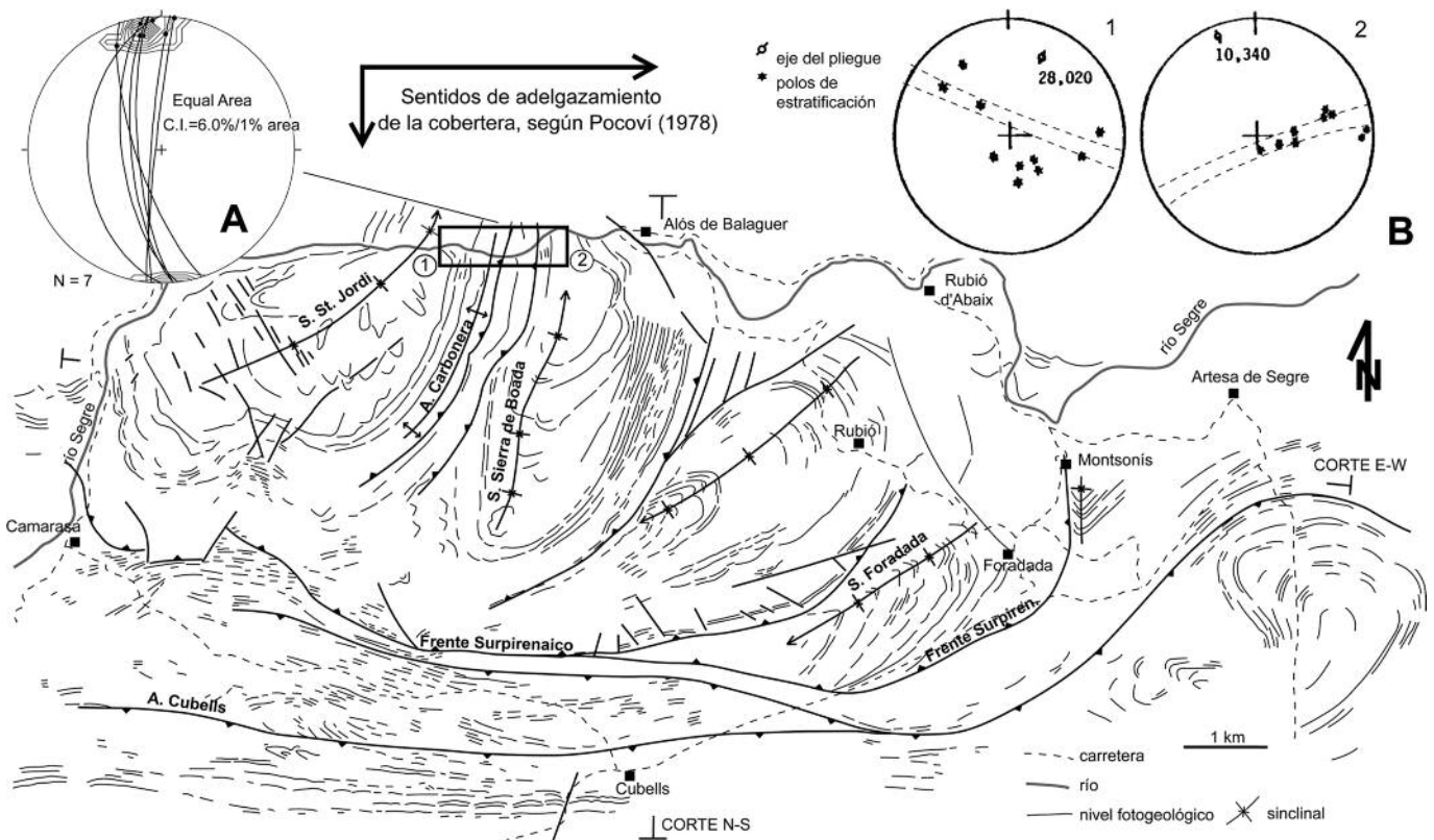
Fig. 2.- Esquema fotogeológico de los pliegues oblicuos de la terminación oriental de las Sierras Marginales y datos estructurales. A) Indicadores cinemáticos (estrias) sobre planos de estratificación. B) Eje de los sinclinales de (1) St. Jordi y (2) Sierra Boada a partir de polos de estratificación. Se observa el carácter no cilíndrico de los mismos.
