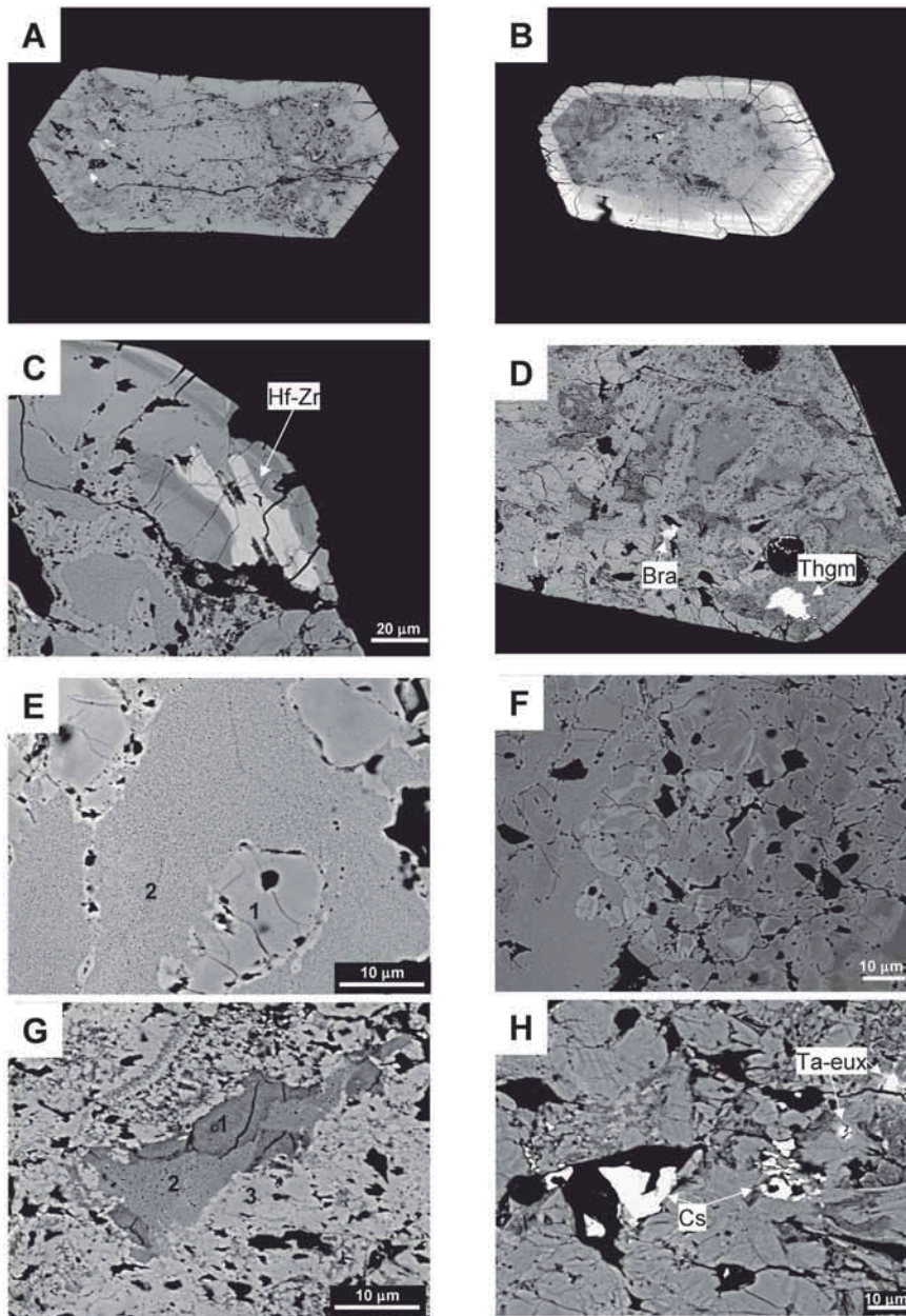
Fig. 2.- Imágenes de electrones retrodispersados mostrando: A) Cristal de circonio (0,9 mm de largo) con zonación pobre. La parte gris oscura en el núcleo corresponde al circonio original metamixto y alterado. La parte clara está recrystalizada y presenta contenidos en Hf similares a la corona. Los puntos brillantes corresponden a inclusiones de thorogumita y tantaexenita. B) Cristal complejo de circonio (0,7 mm de largo). El núcleo es texturalmente heterogeneo. La corona presenta zonación oscilante y contenidos en HfO 2 de hasta el 34 % en peso. C) Borde de un cristal mostrando evidencias de recrystalización a favor de microfisuras y la inclusión de un microcristal de circonio con alto contenido en Hf. D) Detalle de un cristal de circonio. En el núcleo se observan texturas pseudocoloformes relacionadas con recrystalización hidrotermal. Thgm: thorogumita; Bra: brabantita. E) detalle del núcleo de un circonio mostrando: 1) relictos del circonio original y 2) textura porosa del circonio metamictico. F) Recrystalización en el núcleo de un circonio. Los microcristales más claros presentan contenidos en Hf similares a los de la corona. G) Detalle en el núcleo de un circonio en que se observan tres etapas: 1) circonio original, 2) circonio metamixto y 3) recrystalización hidrotermal de circonio. H) Núcleo de un cristal con inclusiones de casiterita (Cs) y tantaexenita (Ta-eux).
