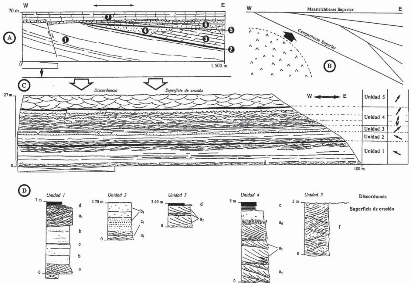
Fig. 2.- A) Corte geológico simplificado de la cantera de Laño (modificado de Gómez-Alday et al. , 1994). 1: Sistema fluvial inferior de cantos «disk shaped». 2: Sistema palustre inferior. 3: Sistema palustre intermedio. 4: Sistema fluvial intermedio. 5: Sistema palustre superior. 6: Sistema fluvial superior. 7: Sistemas litorales superiores. B) Esquema de la disposición de las discordancias angulares sobre el área de levantamiento diapírico. C) Diagrama de facies del Sistema fluvial inferior de cantos «disk shaped» en la pared W de la cantera de Laño. Las flechas indican los valores medios de las paleocorrientes medidas. D) Columnas estratigráficas detalladas de cada unidad. Descripción de las facies en el texto.
