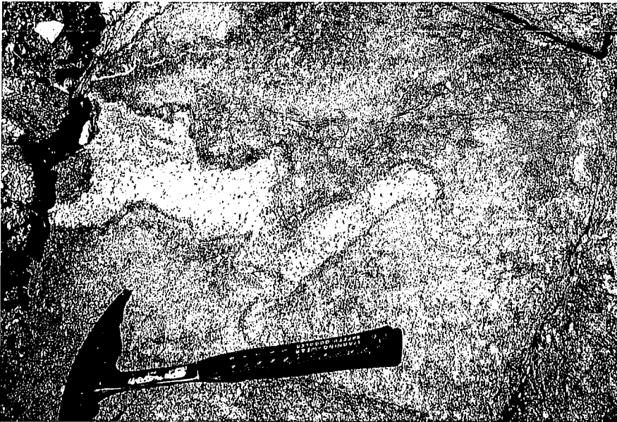
Fig.4.- Deformación plástica e hibridismo de la cuarzodiorita y la granodiorita.
