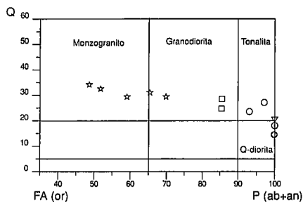
Fig. 2.- Clasificación modal QAP mesonormativa de las rocas de Sant Esteve. (Strecksien, 1976). (Norma bi-hb; FeO/(FeO+Fe2O3) = 1; NewPet 1994, Univ. Newfoundland). Leyenda: estrellas: intrusión granítica tardía; cuadrados: granodioritas del complejo; círculos: enclaves de grano fino; triángulo: masas de grano medio; rombo: dique sin-plutónico.
