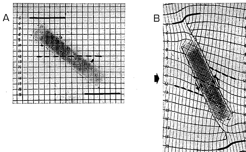
Fig. 2.—Estadios inicial (A) y final (B) del experimento realizado (38% de acortamiento), donde se resaltan los marcadores de la malla analizados.
