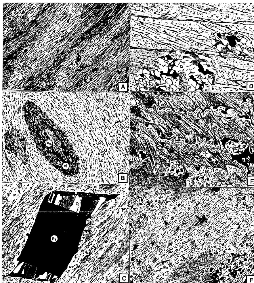
Fig. 3.—Microestructuras asociadas a la esquistosidad. A: Orientación preferente de filosilicatos (Agregados clorita-mica y micas). B: Vacuolas de minerales cloríticos. C: Zonas abrigadas. D: Planos de disolución-acumulación, rectilíneos. E: Pseudocrenulación en calizas limosas finamente laminadas. F: Orientación preferente de filosilicatos en una arenisca con «rough cleavage».
