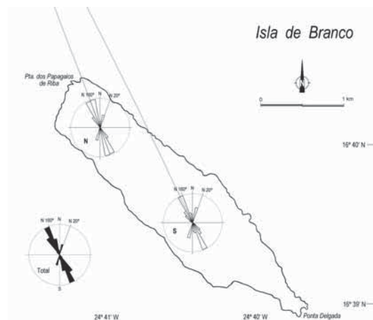
Fig. 6.- Diagrama de distribución de diques, para el conjunto de la isla (total) y las estaciones Norte (N) y Sur (S). En cada diagrama se indica entre paréntesis el número de medidas. Las líneas de prolongación de las direcciones dominantes medias convergen ligeramente hacia el posible centro del edificio primitivo.
