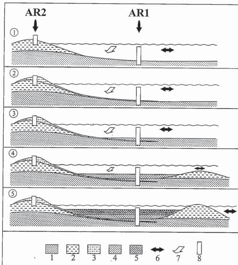
Fig. 2.- Evolución del sector de Las Nuevas (Parque Nacional de Doñana). Leyenda: 1: depósitos de lagoón (arcillas); 2: depósitos de levee (arcillas); 3: chenier (arcillas limosas); 4: depósitos de transición (arcillas); 5: depósitos de laguna (arcilla); 6: influencia mareal; 7: influencia fluvial; 8: sondeos estudiados.
