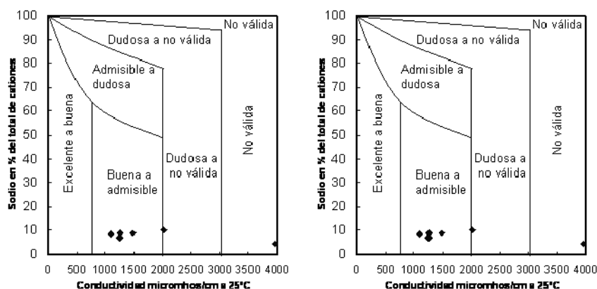
Fig. 5. Representación de los Diagramas de L.V. Wilcox para las aguas drenadas de los Tratamientos Agua Destilada y SFM3 (arriba y abajo respectivamente).
