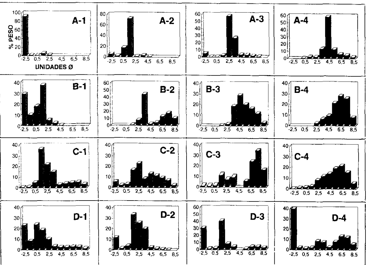
Fig. 4.—Distribuciones granulométricas más frecuentes de las litofacies estuarias de la costa de Huélfva. Las letras representan una disminución desde A hacia D en la clasificación de las partículas del sedimento y los números (1 a 4) la disminución del tamaño de grano medio.
