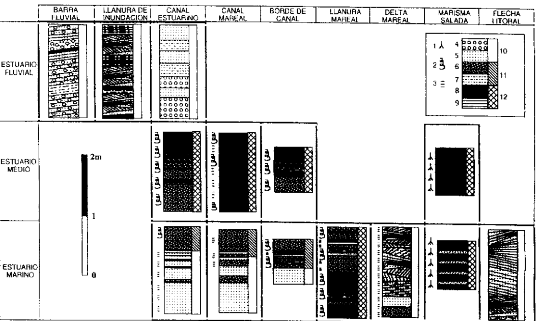
Fig. 3.—Síntesis de las facies deposicionales de la costa de Huelva con indicación de los sectores estuarinos en que aparecen. 1: bioturbación por raíces; 2: bioturbación animal; 3: conchas y fragmentos de conchas; 4: gravas; 5: arenas limpias; 6: arenas fangosas; 7: limos; 8: fangos; 9: laminación s.l.; 10: bioturbación ausente; 11: bioturbación escasa; 12: bioturbación intensa.
