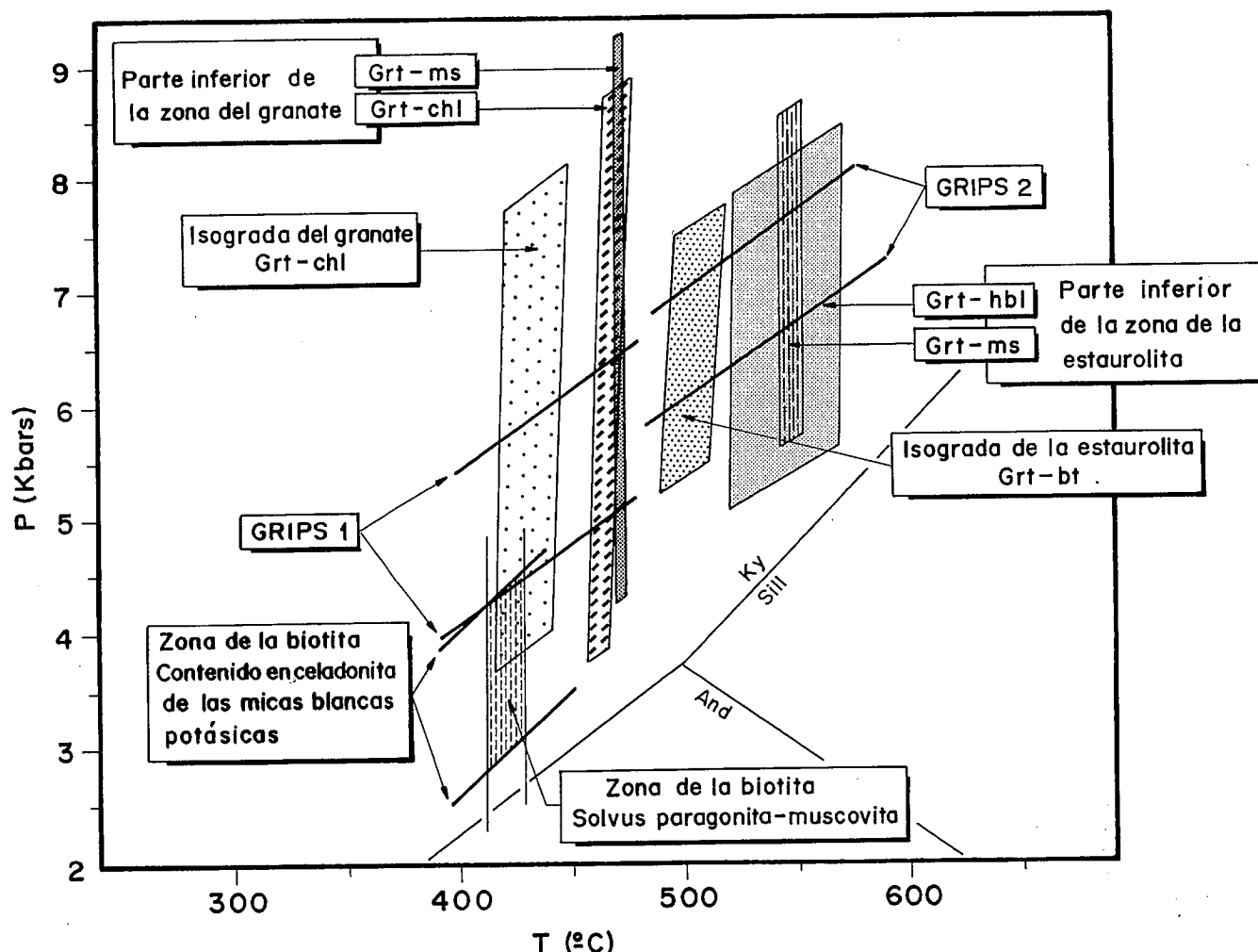
Fig. 2.- Diagrama P-T mostrando los resultados termobarométricos obtenidos para las asociaciones metamórficas sin - D_2 de las zonas de la biotita, granate y estaurolita de las formaciones de El Broumi - Ouled Hassine y de Lalla Tittaf. Las estimaciones P-T en la zona de la biotita han sido realizadas con termometría de exolución paragonita - muscovita (Eugster et al. , 1972) y con barometría basada en el contenido en celadonita de las micas blancas potásicas (Massone y Schreyer, 1987). En las metabasitas, la temperatura ha sido calculada mediante el termómetro grt - hbl (Graham y Powell, 1984). El barómetro GRIPS ha sido aplicado en la zona del granate (1) y en la de estaurolita (2). El resto de las abreviaturas son como en la Fig. 1.
