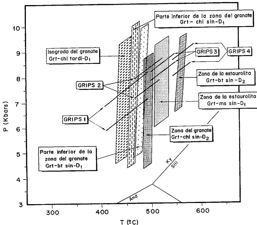
Fig. 1.- Diagrama P - T mostrando los resultados termobarométricos obtenidos para las asociaciones metamórficas sin - D 1 y sin - D 2 de las zonas del granate y de la estauroлита de la Formación de Skhour. Termómetros: grt - chl (Ghent et al. , 1987); grt - bt (Ferry y Spear, 1978; Hodges y Spear, 1982; Hoinkes, 1986); grt - ms (Hynes y Forest, 1988). Barómetro GRIPS (Bohlen y Liotta, 1986): 1 y 2, asociaciones sin - D 1 y sin - D 2 , respectivamente, de la zona del granate; 3 y 4, asociaciones sin - D 1 y sin - D 2 , respectivamente, de la zona de la estauroлита. Límites de estabilidad de los polimorfos de silicato aluminico, según Holdaway (1971). Abreviaturas minerales según Kretz (1983).
