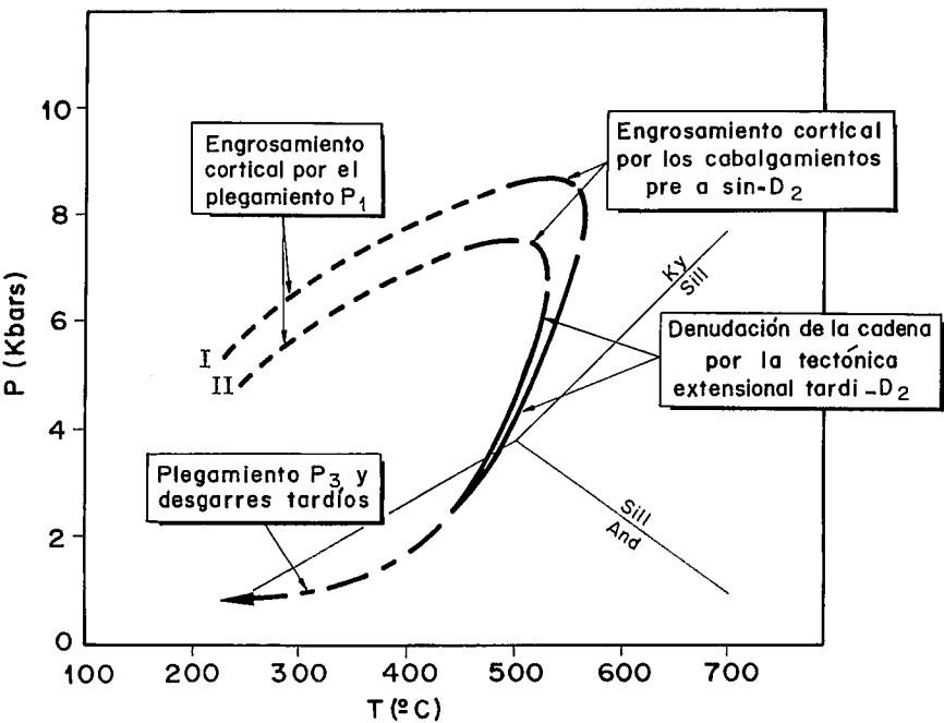
Fig. 3.- Trayectorias P - T estimadas para las litologías de la zona de la estauroлита de la Formación de Skhour (I) y de las formaciones de El Broumi - Ouled Hassine y de Lalla Tittaf (II). En el caso de las formaciones de Rehamna Oriental (II), el recorrido sin - D 1 de la trayectoria ha sido supuesto.
