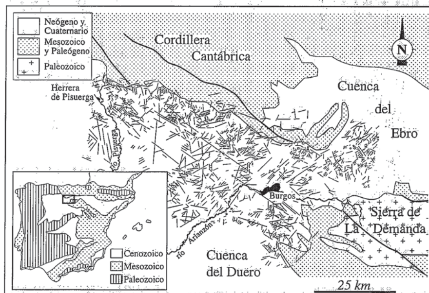
Fig. 1- Esquema geológico del sector estudiado y cartografía de lineamientos obtenidos a partir del estudio de la imagen de satélite.
