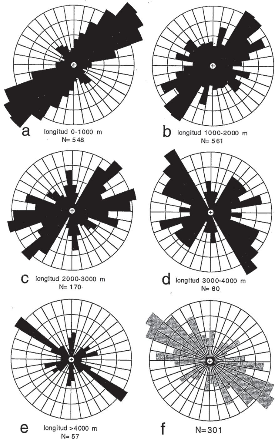
Fig. 3- a, b, c, d, e) Diagramas en rosa que muestran la distribución de orientaciones en función de la longitud de los lineamientos. f) Orientaciones de las principales estructuras cartográficas que afectan al substrato pre-neógeno. (Círculo externo: 10% de los datos).
