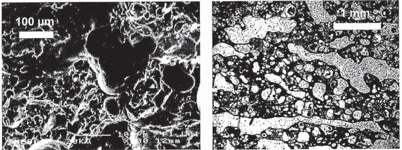
Fig. 1.- Imágenes de microscopio electrónico de barrido y microscopio petrográfico del vidrio vesicular de la roca pumícea de El Gasco.
