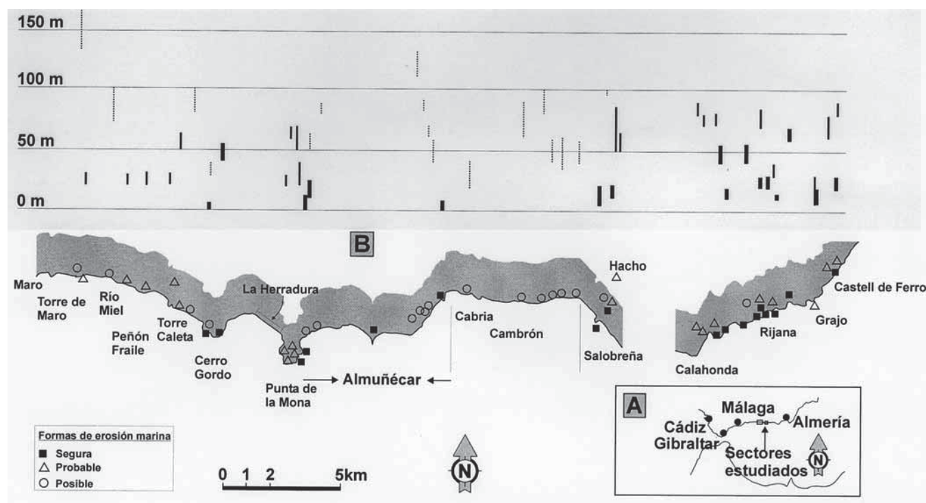
Fig. 1.- A.- Situación general del área estudiada. Se marca la posición de B. B.- Situación de las distintas formas de abrasión marina existentes entre Maro y Castell de Ferro. La alturas de cada una de ellas se muestra encima, así como si es una forma segura, probable o simplemente posible (líneas gruesas, finas y a puntos respectivamente).
