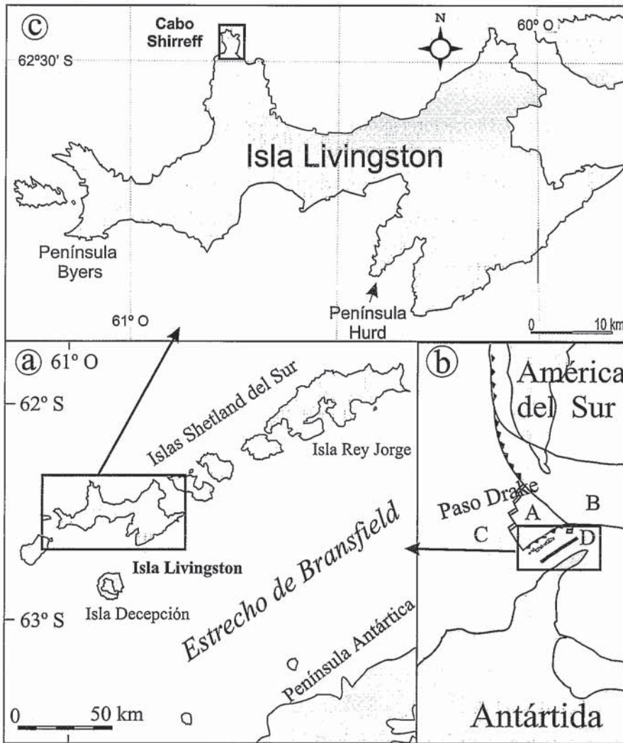
Fig. 1.- a: Situación geográfica de las Islas Shetland del Sur. b: Esquema tectónico regional. A = Placa Drake, B = Placa Sandwich, C = Placa Antártica, D = Cuenca de Bransfield. c: Situación del área de estudio.
