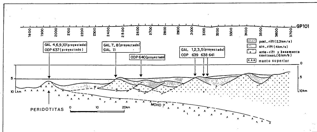
Fig. 2.—Corte esquemático del Margen de Galicia en la línea sísmica GP 101 (Uns. Fr. du Pétrole). S, «reflector S».
