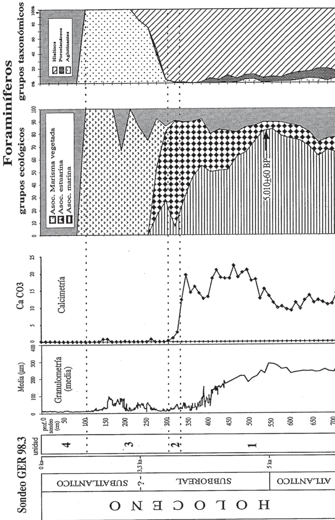
Fig. 2.- Evolución de los parámetros microfauunísticos y sedimentológicos estudiados en el sondeo holoceno GER 98.3. Se muestra la distribución de las asociaciones de foraminíferos bentónicos (marinas, estuarinas y de marisma) y los tipos morfológicos (hialinos = Miliolina, porcelanáceos = Rotaliina, aglutinantes = Textularina) más característicos, así como las granulometrías y calcimetrías de las cuatro unidades diferenciadas.
