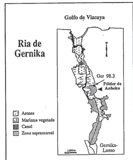
Fig. 1.- Localización del sondeo estudiado (Ger 98.3).
