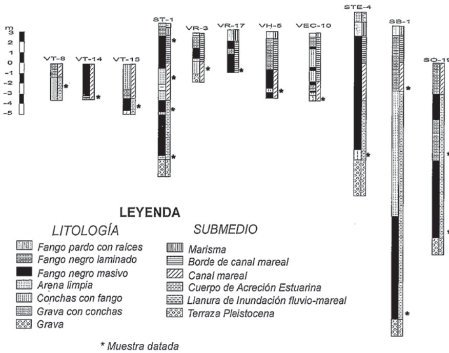
Fig. 2.- Columnas litológicas de los testigos estudiados y localización de las muestras datadas con 14 C.
