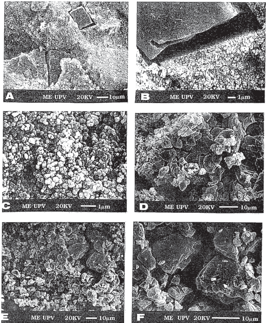
Fig. 2.- Ultrafacies al microscopio electrónico de barrido (SEM) de los nódulos de sílex modificados. (A) Cristales de microcuarzo, como principal constituyente del nódulo, con romboedros de dolomita (Zona A, Formación de Ribera Alta, muestra no atacada con HF). (B) Detalle de la anterior fotografía. Se aprecia una disolución tardía de los bordes de dolomita y un nudo contacto planar con los microcuarzos sin disolver. (C) Detalle de los cristales de microcuarzo (<0.3mm), con una porosidad intercrystalina importante. (D) Cristales de megacuarzo rodeados de variedades fibrosas de la sílice (Zona B, Formación de Ribera Alta, muestra atacada con HF). (E) Cristales de megacuarzo y microcuarzo con una alta porosidad en los sílex de la Formación de Cueva (muestras no atacadas con HF). (F) Detalle de la anterior fotografía, con pequeñas secciones de dolomita.
