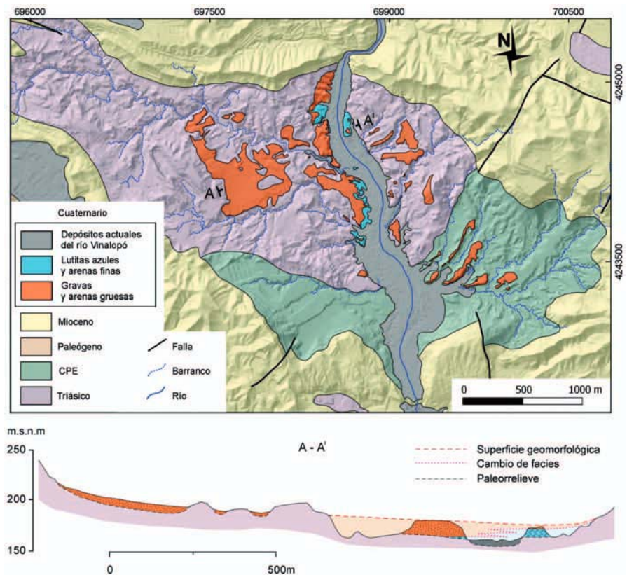
Fig. 2.- Mapa y corte geológico de la zona de estudio. Ver figura en color en la web.
