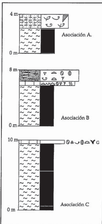
Figura 1.- Asociaciones de facies descritas en la secuencia de depósito Aptiense Inferior.
