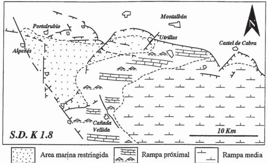
Figura 2.- Mapa paleogeográfico de la S.D. Aptiense inferior en la Subcuenca de Las Parras
