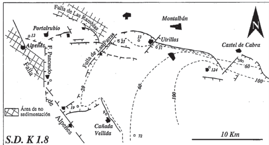
Figura 4.- Mapa de isopacas para la secuencia de depósito Aptiense Inferior en la Subcuenca de Las Parras.
