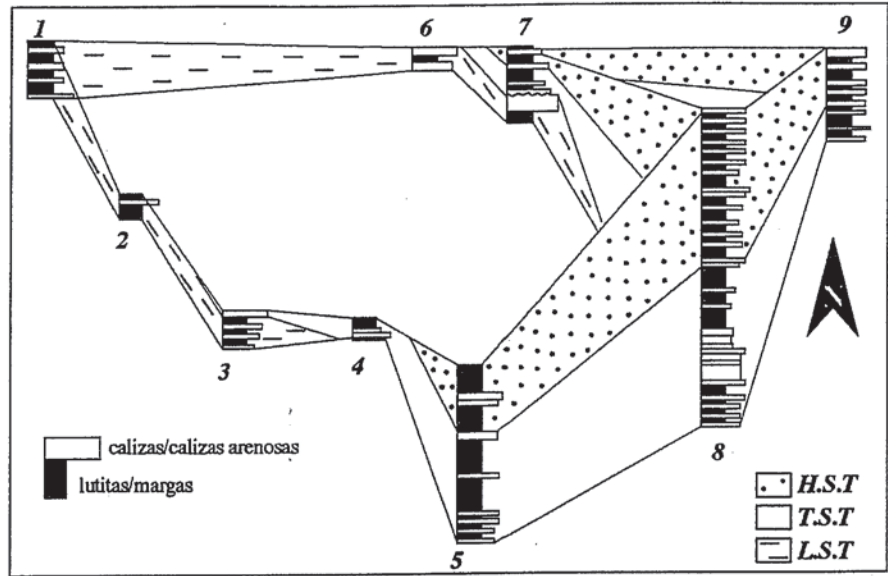
Figura 3.- Panel de correlación y distribución de los cortejos sedimentarios para la secuencia de depósito Aptiense inferior en la Subcuenca de Las Parras. 1. Alpeñes, 2. Pancrudo, 3. Rillo, 4. Cañada Vellida, 5. Galve Norte, 6. Barranco del Cocharro, 7. Utrillas, 8. Palomar de Arroyo y 9. Castel de Cabra.
