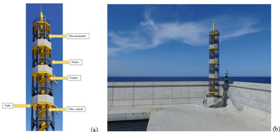
Figura 5. Partes principales de la estructura portante del faro (a). Vistas finales del faro terminado (b). Fuente: Elaboración propia.
