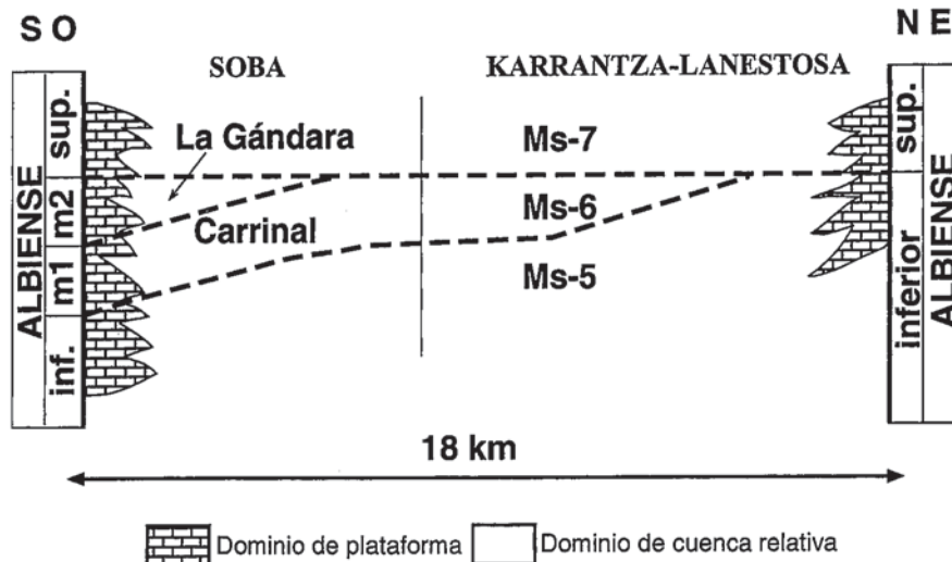
Fig. 2.- Esquema simplificado de correlación de las secuencias del Albiense Medio con representación en plataforma en Soba (Cantabria) y las secuencias equivalentes en la zona de Karrantza. m1: Alb. Medio, parte inferior. m2: Alb. Medio, parte superior. Basado en García-Mondéjar y Fernández-Mendiola (1998), García-Mondéjar, comunicación personal y Ms-5 a Ms-7 en López-Horgue (2000).
