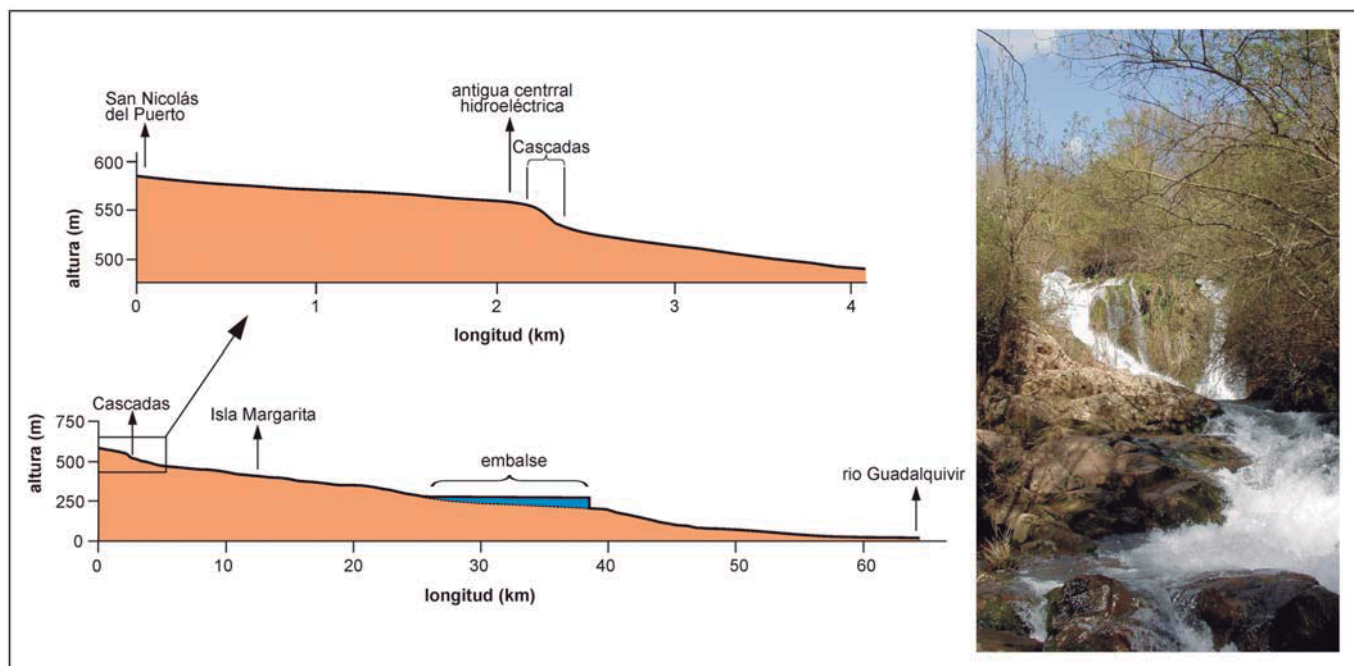
Fig. 2.- Perfil longitudinal de la riera del Huézna y detalle del tramo de las cascadas. La fotografía muestra un aspecto general del salto inferior de las Cascadas del Huézna.
