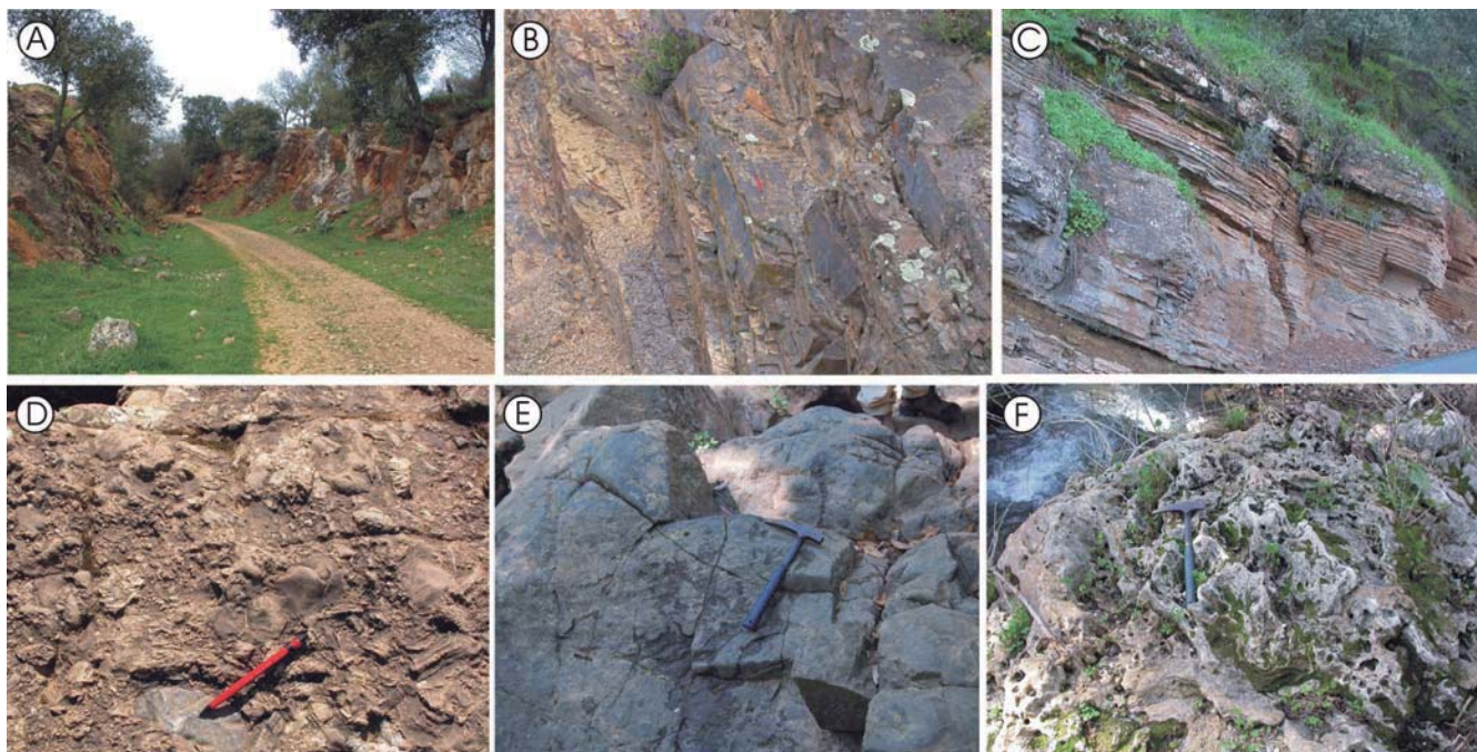
Fig 3.- Aspecto de campo de las rocas del entorno de las Cascadas del Huézna. A, B y C corresponden a afloramientos de rocas de la Formación Capas de Campoallá esencialmente carbonatadas, detríticas y mixtas, respectivamente. D, E y F son fotografías de detalle de la brecha de la falla del Martinete, de la microdiorita del dique asociado a esta misma falla y de depósitos travertínicos recientes.
