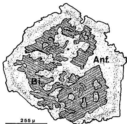
Fig. 1.—Sustitución de cristales de biotita por anfíbol en la roca intrusiva.
