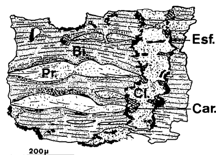
Fig. 2.—Secuencias de transformación en biotitas de la roca intrusiva: 1ª) transformación en prehnita; 2ª) cloritización parcial con carbonatos y esfenas como subproductos.
