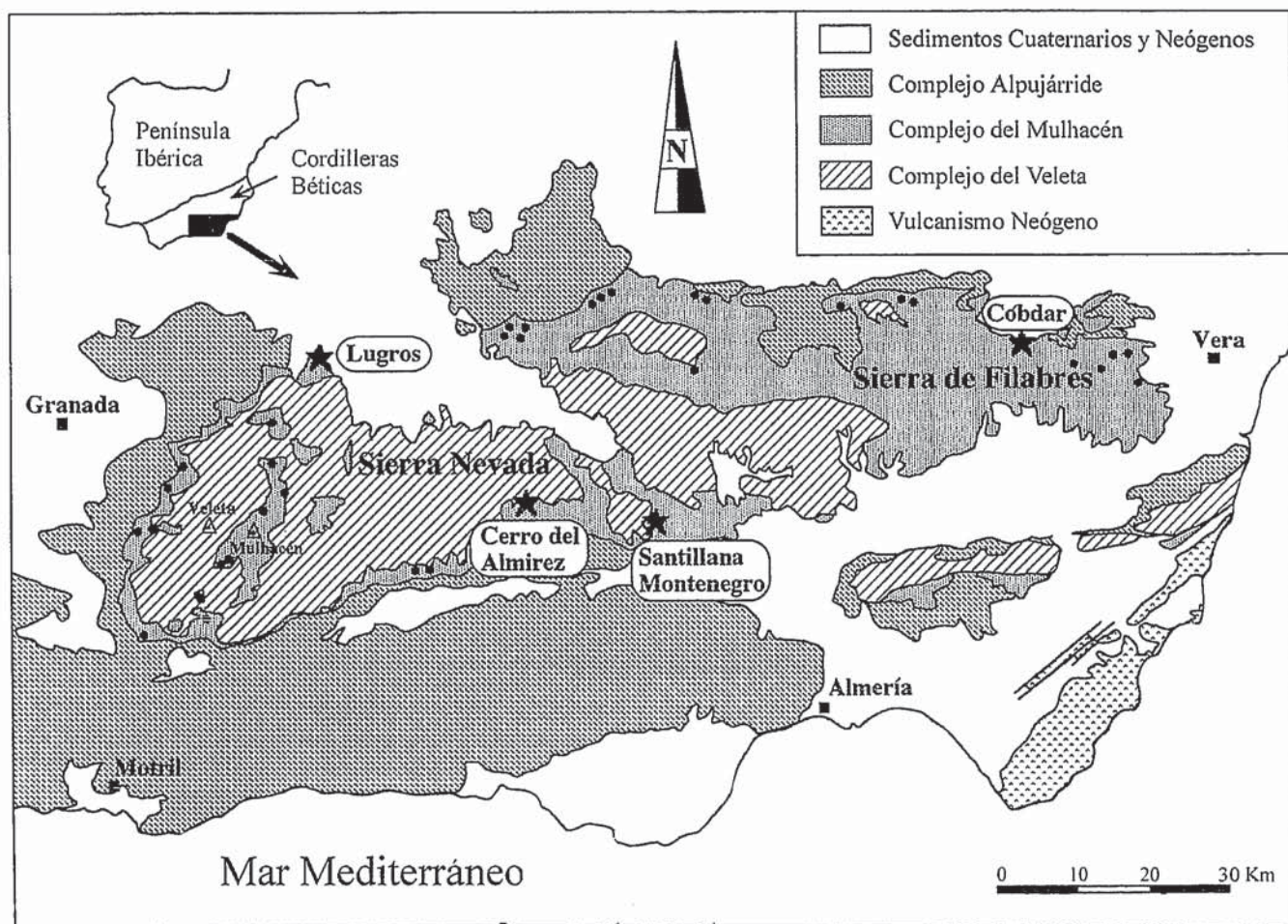
Fig. 1.- Mapa geológico sintético del sector central-oriental de las Cordilleras Béticas. Los puntos negros y estrellas representan los principales afloramientos de la Asociación Ofiolítica Bética.
