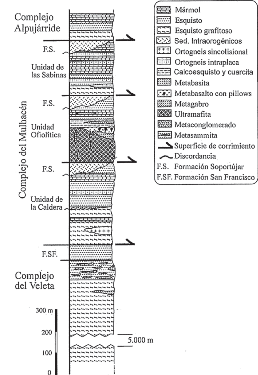
Fig. 2.- Columna litostratigráfica sintética de los complejos del Veleta y Mulhacén, junto con una litostratigrafía simplificada (sin escala) del Complejo Alpujarride.
