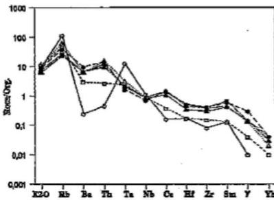
Fig. 3.1.— Diagrama de variación multielementos traza (Diagrama Spider) de Pearce et al., (1984).
