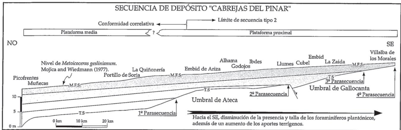
Fig. 2.- Cuadro esquemático que muestra la situación de los perfiles, distribución de las parasecuencias, rasgos paleogeográficos y principales características de la secuencia de depósito «Cabrejas del Pinar».
