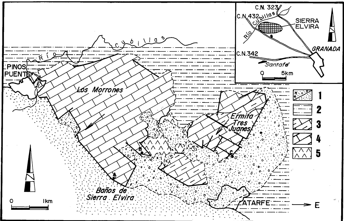
Fig. 1.- Situación geográfica y esquema hidrogeológico de Sierra Elvira. 1: Conglomerados arcillosos cuaternarios de pie de monte (acuitardo)/Gravas, arenas y limos aluviales (acuífero); 2: Conglomerados arcillosos y arcillas del Pliocuatnario (acuitardo); 3: Margocalizas y calizas margosas del Jurásico (acuitardo); 4: Dolomías y calizas, con eventuales tramos margocalizos, del Jurásico (acuífero de Sierra Elvira); 5: Margas con yesos del Triás (acuícludo); A: Baños de Sierra Elvira; B: Sima de Raja Santa; C: Sondeo del Ayuntamiento de Atarfe; E: Dirección del flujo. Adaptado del IGME (1988).
