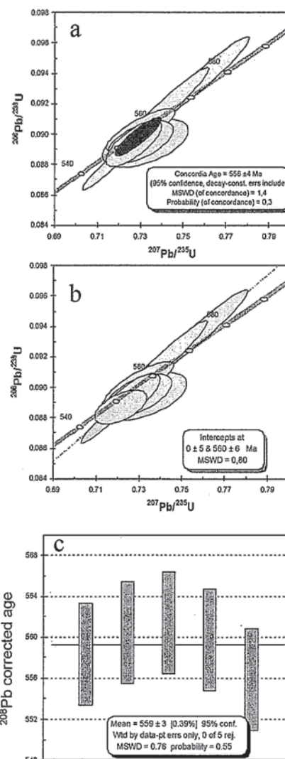
Fig. 3.- A) Diagrama de concordia de Wetherill de los análisis de la Tabla 1. La elipse oscura representa la edad de concordia (Ludwig, 1998) de los 8 análisis. Las elipses representan los errores 2\sigma . B) Diagrama de concordia de Wetherill mostrando la edad de intersección de una discordia forzada a través de 0 \pm 5 Ma. C) Media ponderada de las edades con el contenido en ^{208}\text{Pb} corregido (Ludwig, 2001) de los circones más concordantes (detalles en el texto).
