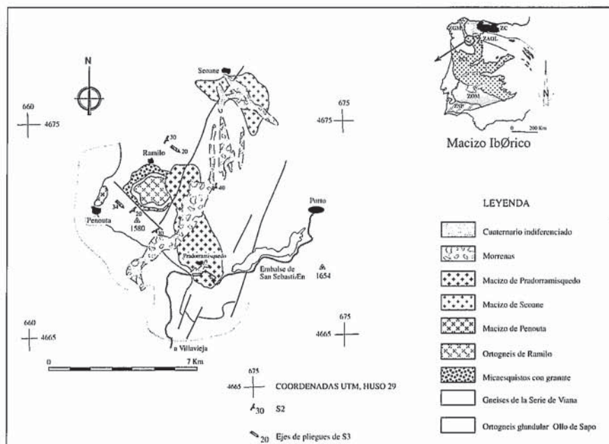
Fig. 1.- Esquema geológico del Macizo de Pradorramisquedo
