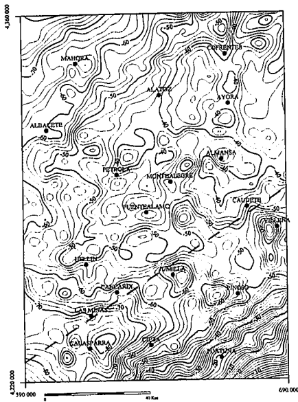
Fig. 2 - Mapa de anomalías gravimétricas de Bouguer. Coordenadas U.T.M. Isolinías 2 mGals. Los trazos discontinuos indican la posición de la estructura de fractura más importante en la zona (Falla de Jumilla).
