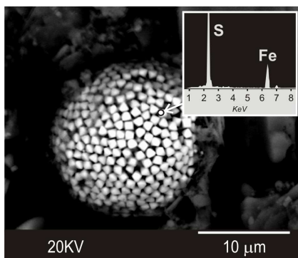
Fig. 2. Imagen de SEM de los sulfuros neoformados encontrados en el contacto con la marisma.
