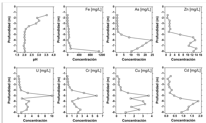
Fig. 1. Evolución con la profundidad del pH y de la concentración de los principales contaminantes en el agua de poro de las muestras de fosfoyeso. A los 8 metros se encuentra el basamento de marisma salada.
