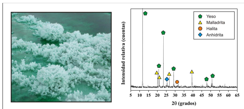
Fig. 3. Fotografía de las eflorescencias que tapizan la superficie de la balsa en época seca así como un análisis ejemplo de DRX.
