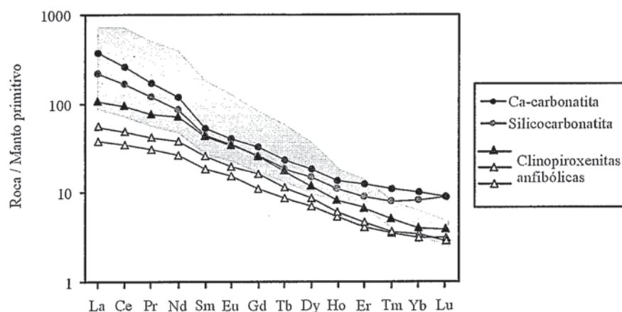
Fig. 3.- Espectros de tierras raras de las clinopiroxenitas y carbonatitas de la asociación alcalino-carbonatítica de Montaña Blanca-Miloch. La similitud entre las pautas indica la existencia de una estrecha relación genética entre ambos tipos petrográficos ultramáficos, así como entre ellos y las carbonatitas de esta asociación. El área sombreada corresponde al campo de variación de los tipos clinopiroxeníticos con perovskita. Datos normalizados según Sun y McDonough (1989).
