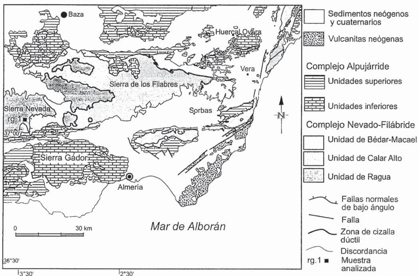
Fig. 1.- Esquema geológico del sureste de las Béticas, incluyendo localización de la muestra estudiada.
