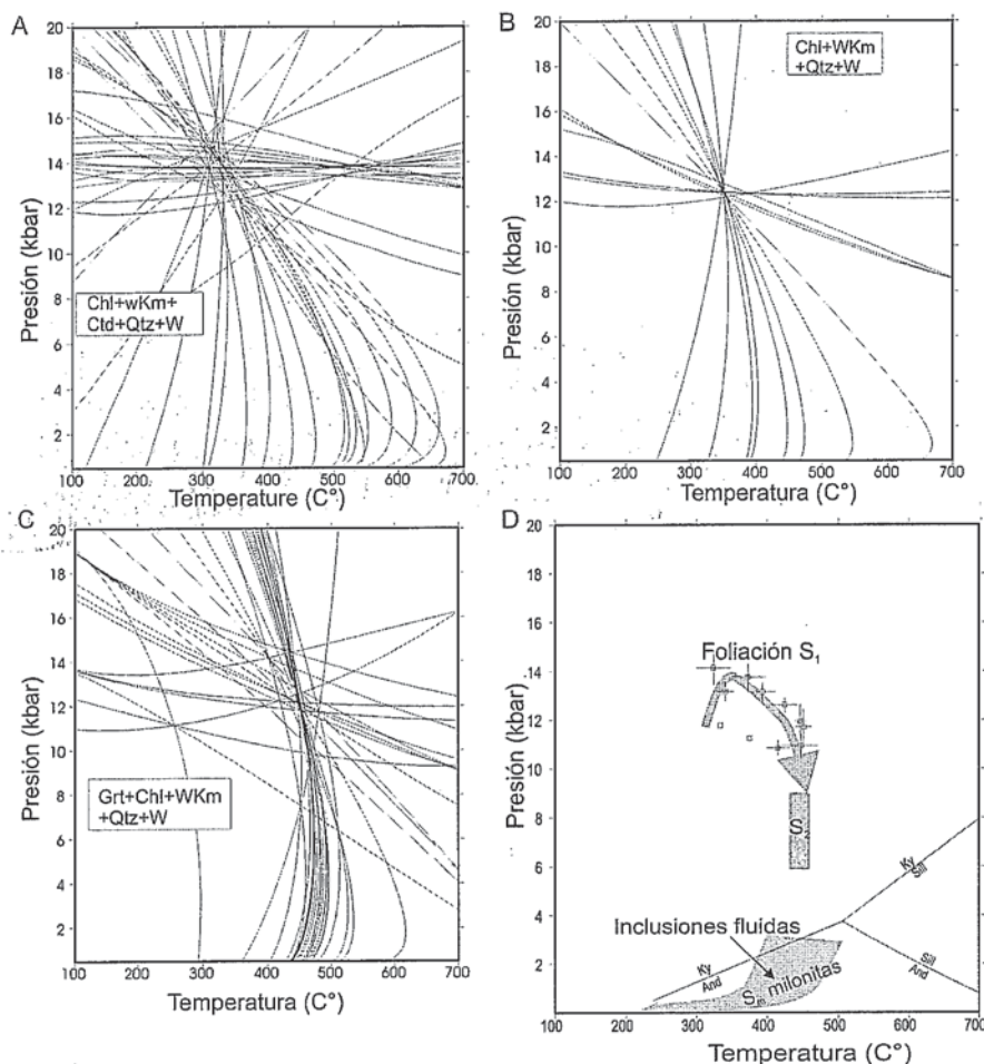
Fig. 2.- Ejemplos de diagramas TWEQU obtenidos para los equilibrios locales estudiados en la muestra rg.1: a) resultado para la paragénesis clorita + fengita + cloritoide + cuarzo + agua, b) equilibrio entre clorita + fengita + granate + cuarzo + agua, c) equilibrio entre clorita + fengita + cuarzo + agua. D) Trayectoria P-T de la unidad de Ragua: foliación S_1 , resultados de este trabajo, foliación S_2 según Martínez-Martínez (1986) y de Jong (1993); trayectoria retrógrada determinada por inclusiones fluidas (González-Casado et al., 1995).
