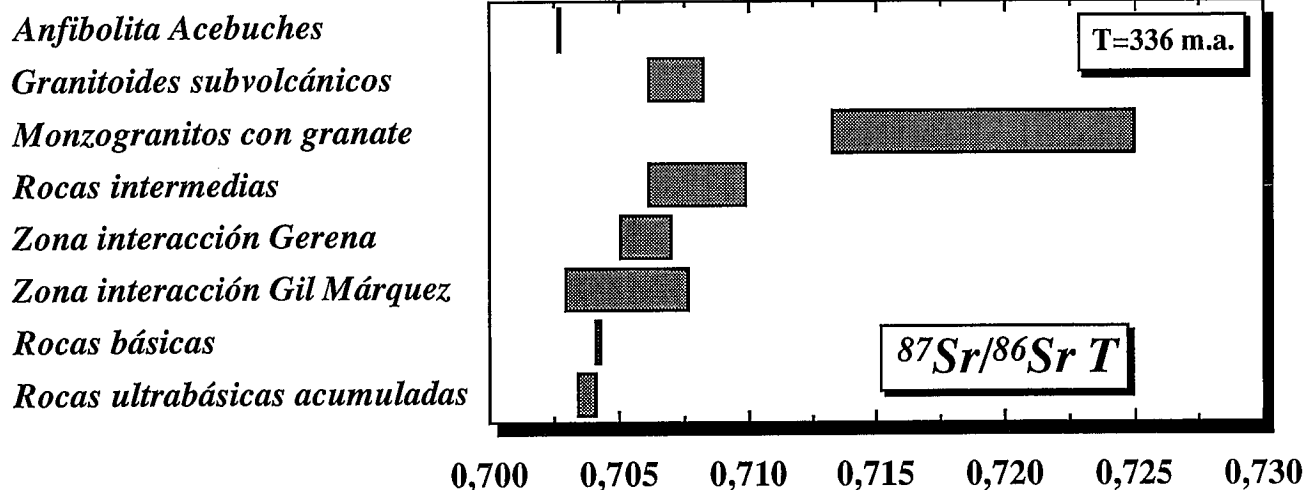
Fig. 4.—Rangos de variación de las relaciones isotópicas iniciales de ^{87}\text{Sr}/^{86}\text{Sr} ( T=336 \text{ m.a.} ) del BSNS.
