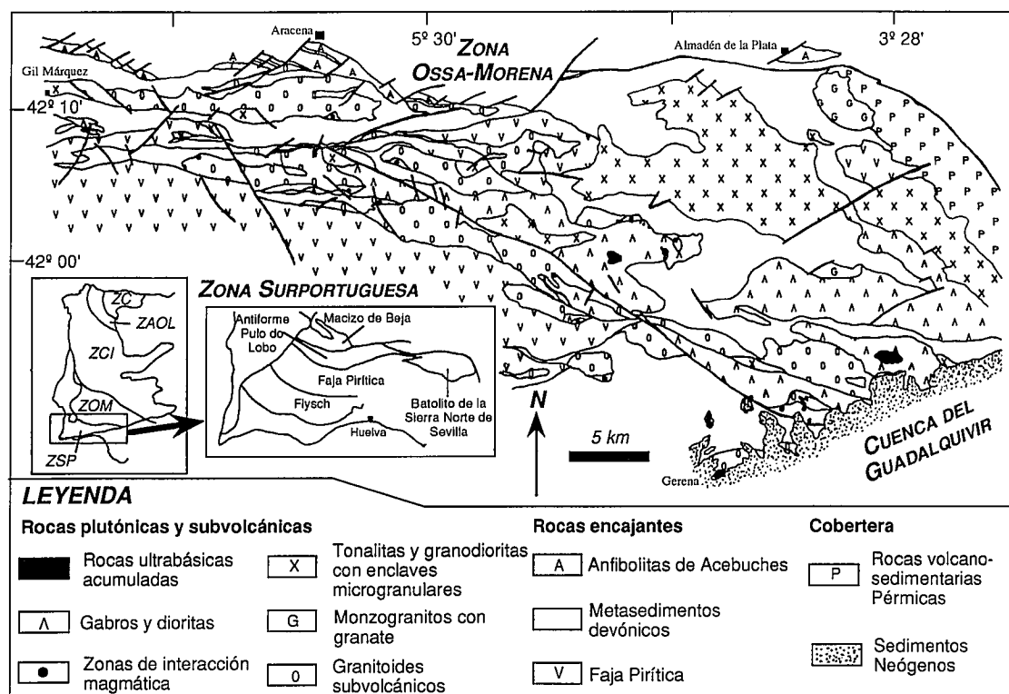
Fig. 1.-Esquema geológico del batolito de la Sierra Norte de Sevilla (BSNS). División de zonas tectónicas del Macizo Ibérico según Julivert et al. (1974)
