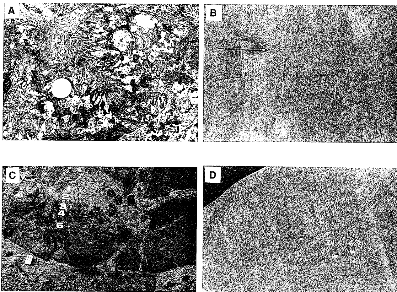
Fig. 2. —A) Gabro pegmatoide con textura gráfica en el contacto entre rocas acumuladas y básicas. B) Gabro anortositico bandeado con laminación paralela y truncada. C) Dique simplutónico del Macizo de Gerena donde se observa un contacto gradual desde el granitoide encajante (I-1 y I-2) a la tonalita de tamaño de grano fino (I-4 y I-5) a través de una tonalita híbrida (I-3). D) Tonalita híbrida con (G-20) y sin (G-21) fenocristales de plagioclasa del Macizo de Gil Márquez.
