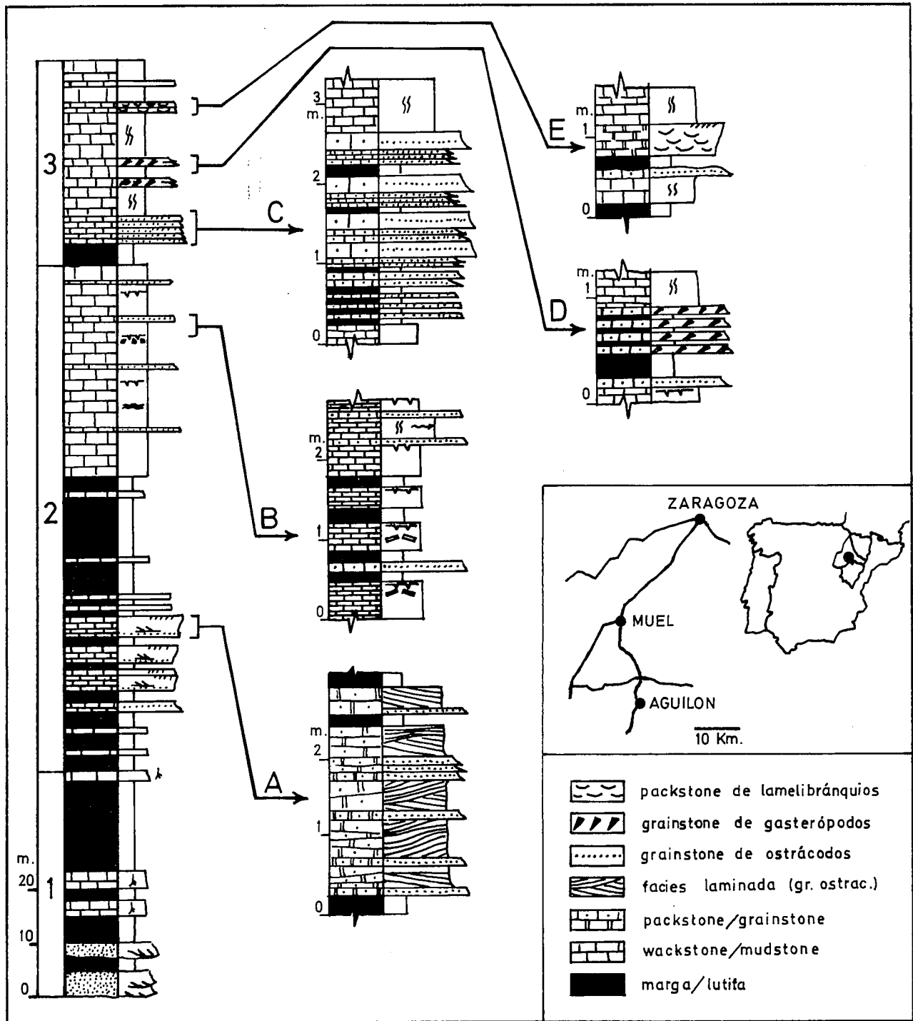
Fig. 1.—Columna general de Aguilón, y detalle de las secuencias estudiadas.
