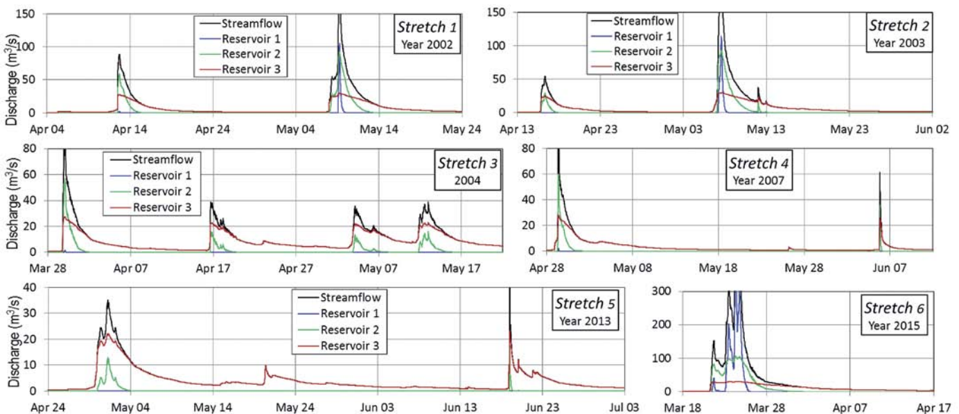
Fig. 4.- Separación de flujo con el modelo 3R, para los seis tramos seleccionados de la serie temporal de la cuenca del río Bergantes. Ver figura en color en la web.
