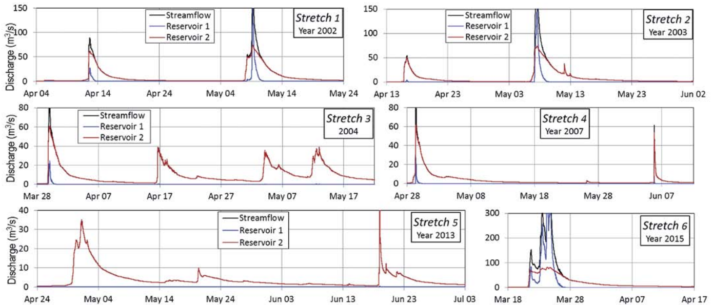
Fig. 3.- Separación de flujo con el modelo 2R, para los seis tramos seleccionados de la serie temporal de la cuenca del río Bergantes. Ver figura en color en la web.
