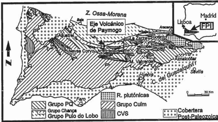
Fig. 1 - Localización geológica del área de estudio en la Faja Pirítica Ibérica (FPI) (Modificada de Carvalho et al., 1976)
