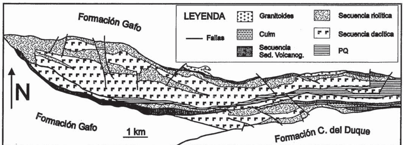
Fig. 2 - Mapa Geológico del eje volcánico de Paymogo
