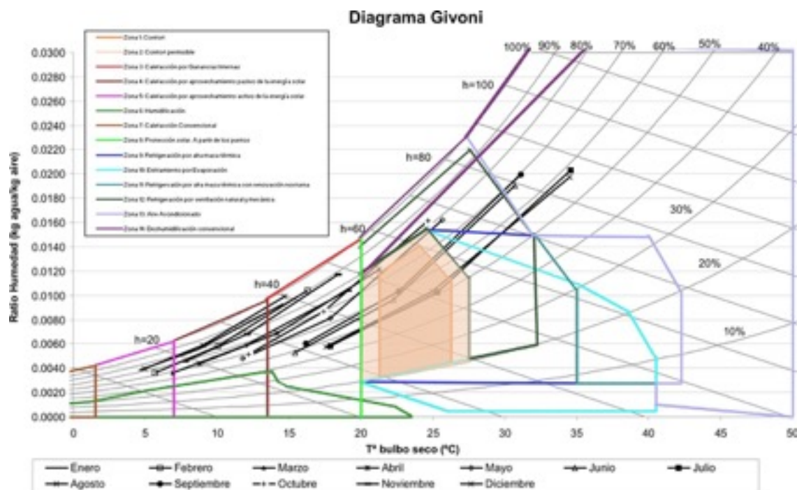
Figura 7. Diagrama sicométrico
