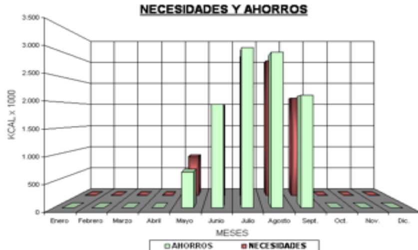
Figura 3: Contribución de los captadores solares térmicos para cubrir las necesidades de refrigeración.
