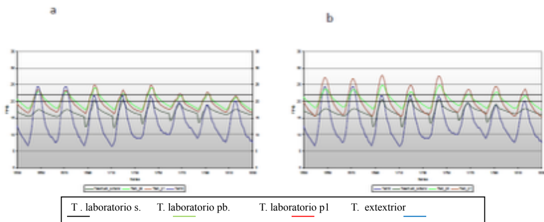
Figura 10: Temperatura en los laboratorios durante el invierno usando a) Cerramiento inercial. b) Cerramiento ligero.
