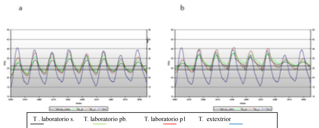
Figura 9: Temperatura en los laboratorios durante el verano usando a) Cerramiento inercial. b) Cerramiento ligero.
