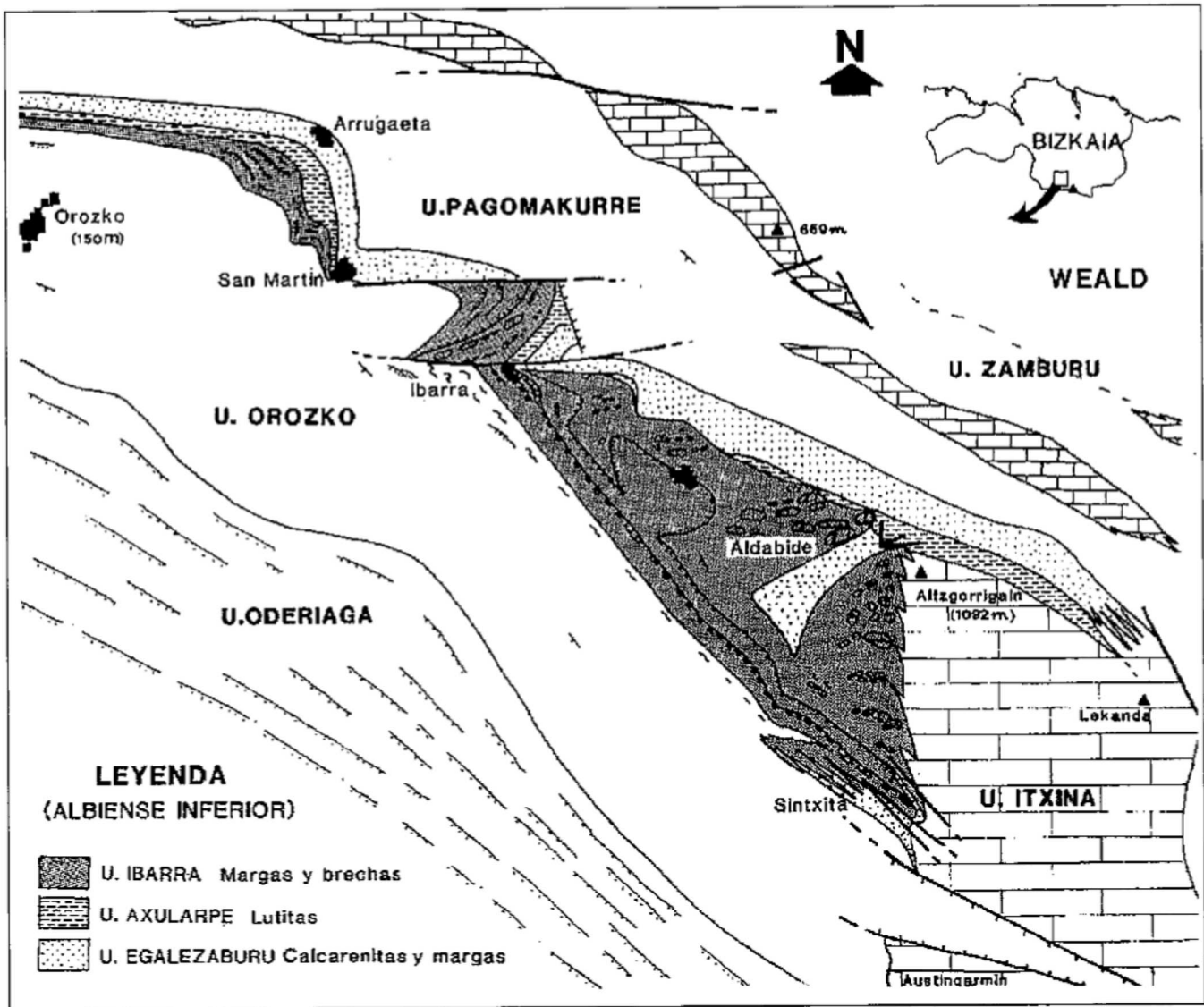
Fig.1.— Mapa simplificado de facies de las unidades del Complejo Urganiano (Zanburu, Pagomakurre, Egalezaburu, Axularpe, Itxina, Ibarra, Orozko, Oderiaga) en el área de estudio.
