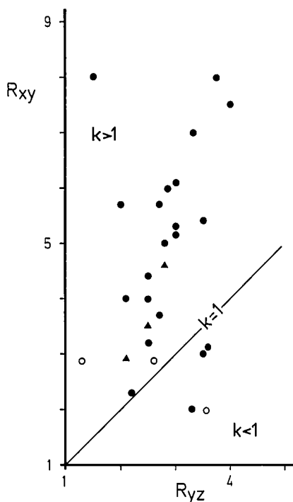
Fig. 3.—Valores de elipticidad en el Ortogneis de Lubrín (Diagrama de Flinn). Este trabajo: puntos rellenos; Borradaile (1976): puntos blancos. Los triángulos representan medidas en conglomerados de la zona de cizalla del Manto de Calar Alto (Jabaloy y González-Lodeiro, 1988).
