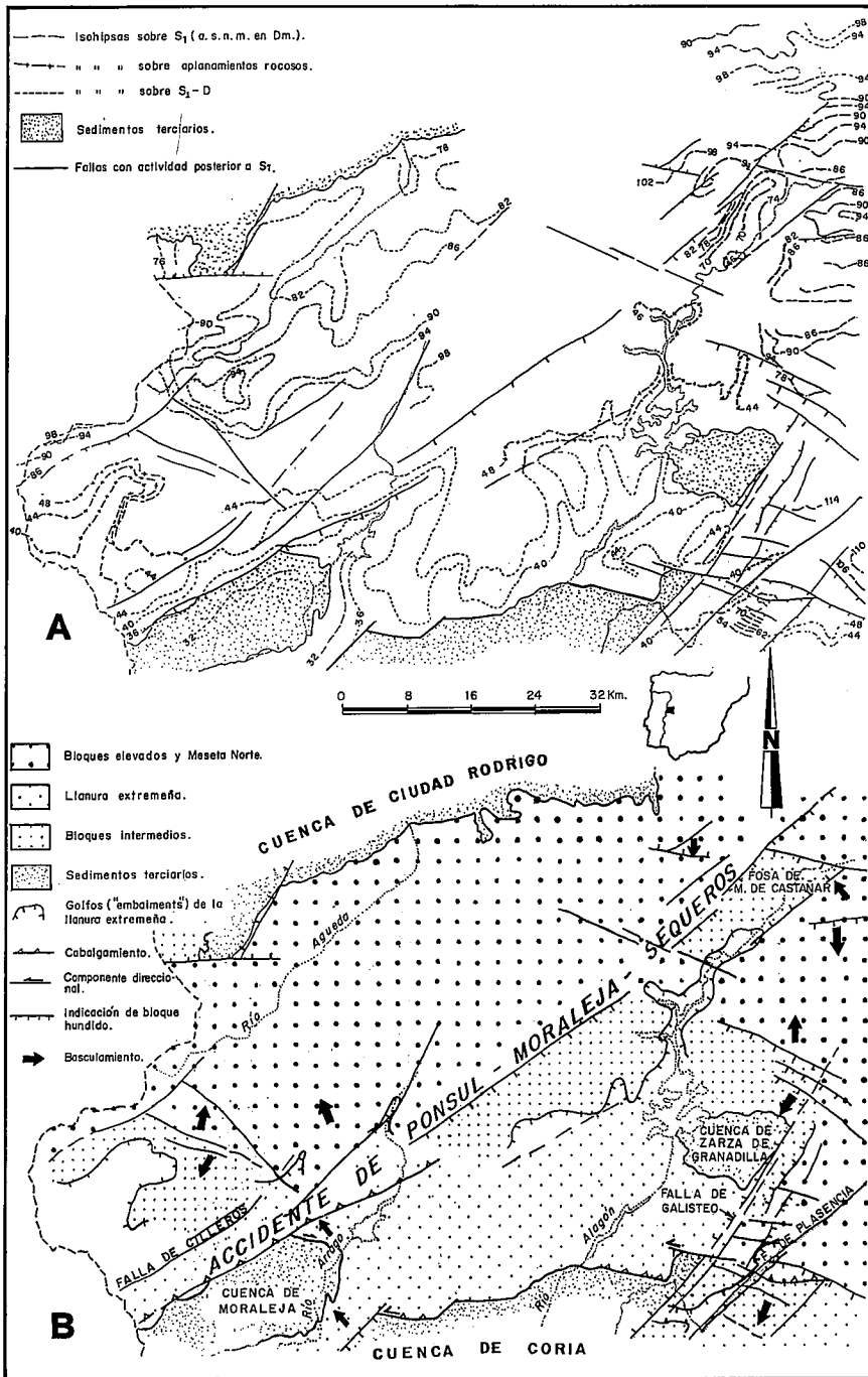
Fig. 1.—A) Los saltos tectónicos en la vertical marcados por las isohipsas de S_1 -D y/o S_1 , son previos a la reelaboración y degradación pliocuaternaria de la superficie paleógena S_1 . Los aplanamientos rocosos, labrados a las cotas de S_1 y/o S_1-D en la llanura extremeña no aparecen desnivelados por fracturas. B) Fallas con actividad alpina y bloques desnivelados tomando como referencia la superficie S_1 .
