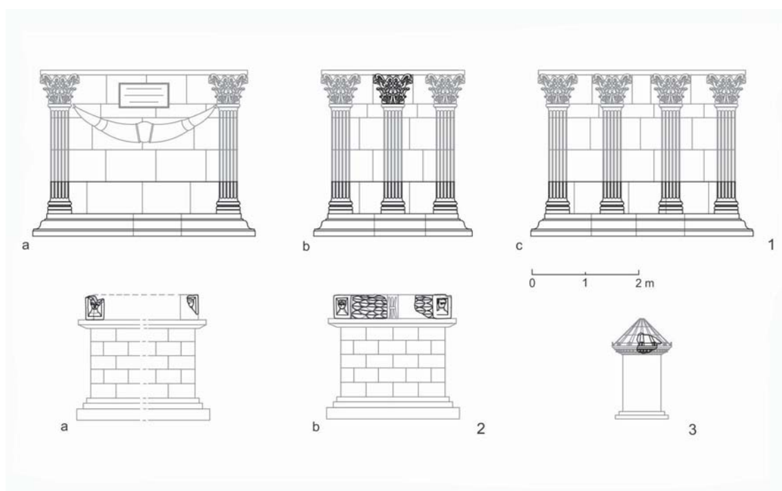
Figura 3. Formas arquitectónicas de los monumentos funerarios identificados en las necrópolis urbanas de Segobriga. 1.- La Tumba Monumental, un posible mausoleo de dos pisos (Cebrián, 2010, fig. 11, 146): a. cara frontal, b. cara lateral, c. cara posterior. 2.- Altar monumental (Noguera, 2012, fig. 64, 356): a. cara frontal, b. cara lateral. 3.- Monumento circular (Trunk, 2015, fig. 6, 330).
