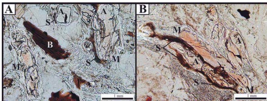
Fig. 2.- Fotomicrografías con luz polarizada paralela, de granitos peraluminicos de Peraleda de San Román (Cáceres), mostrando las relaciones texturales entre andalucita (A), moscovita (M), sillimanita fibrolítica (S) y biotita (B). A) muestra 106809, B) muestra 106810. La andalucita (variablemente pleocroica por presentar zonado químico) aparece envuelta por moscovita y fibrolita. Escala igual a 1 mm. Ver texto para más aclaraciones.
