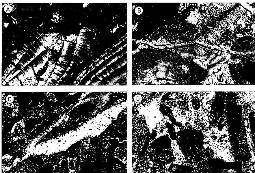
Fig. 1.- Microfotografías de luz transmitida y nícoles paralelos de algunas variedades comerciales del Crema Marfil: A. Estilolito mostrando una superficie de disolución dentada que afecta a un nummulites. Variedad Grano de Arroz. Longitud de la ventana 1 mm. B. Vénula asociada a superficie estilolítica. Variedad Aguas Oscuras. Longitud de la ventana 1 mm. C. Vénulas subparalelas, la mayor muestra relleno politextural. Variedad Crema Marfil Veta. Longitud de la ventana 1 mm. D. Cementación polifásica. Observense los grandes cristales que ocluyen la porosidad interpartícula. Variedad Pintas. Longitud de la ventana 2 mm.
