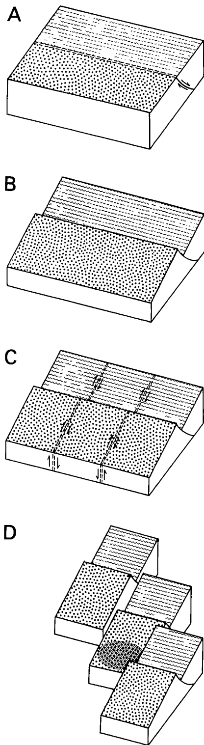
Fig. 2.—Modelo conceptual en el que se recogen las dos etapas de fracturación jurásicas descritas en el texto: A: Lías inferior. B: Carixiense. C: Lías superior-Bathoniense medio. D: Límite Bathoniense medio-superior. A puntos: Unidades tipo Lobatejo-Pollos. A rayas: Unidades tipo Camarena-Lanchares. Area sombreada en fig. D: ámbito de depósito de las brechas estudiadas.
