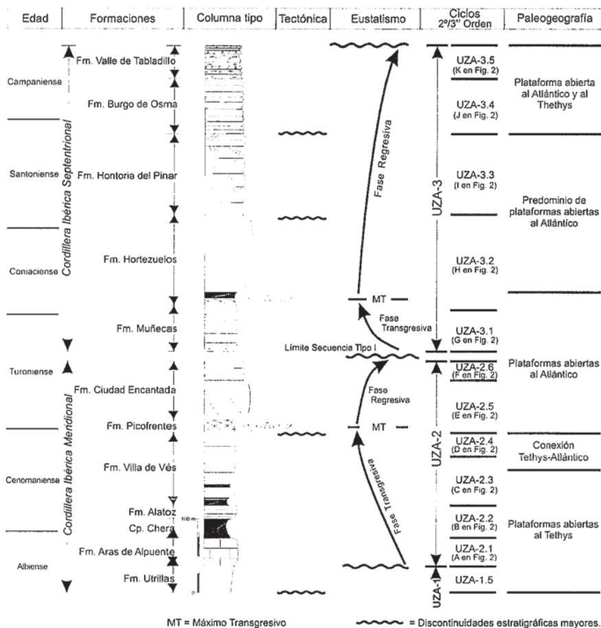
Fig. 1.- Columna sintética del Cretácico superior de la Cordillera Ibérica, relacionando las unidades litoestratigráficas más relevantes, eventos tectónicos, etapas paleogeográficas y ciclos deposicionales de baja frecuencia, referenciados según la nomenclatura de Haq et al. (1988).
