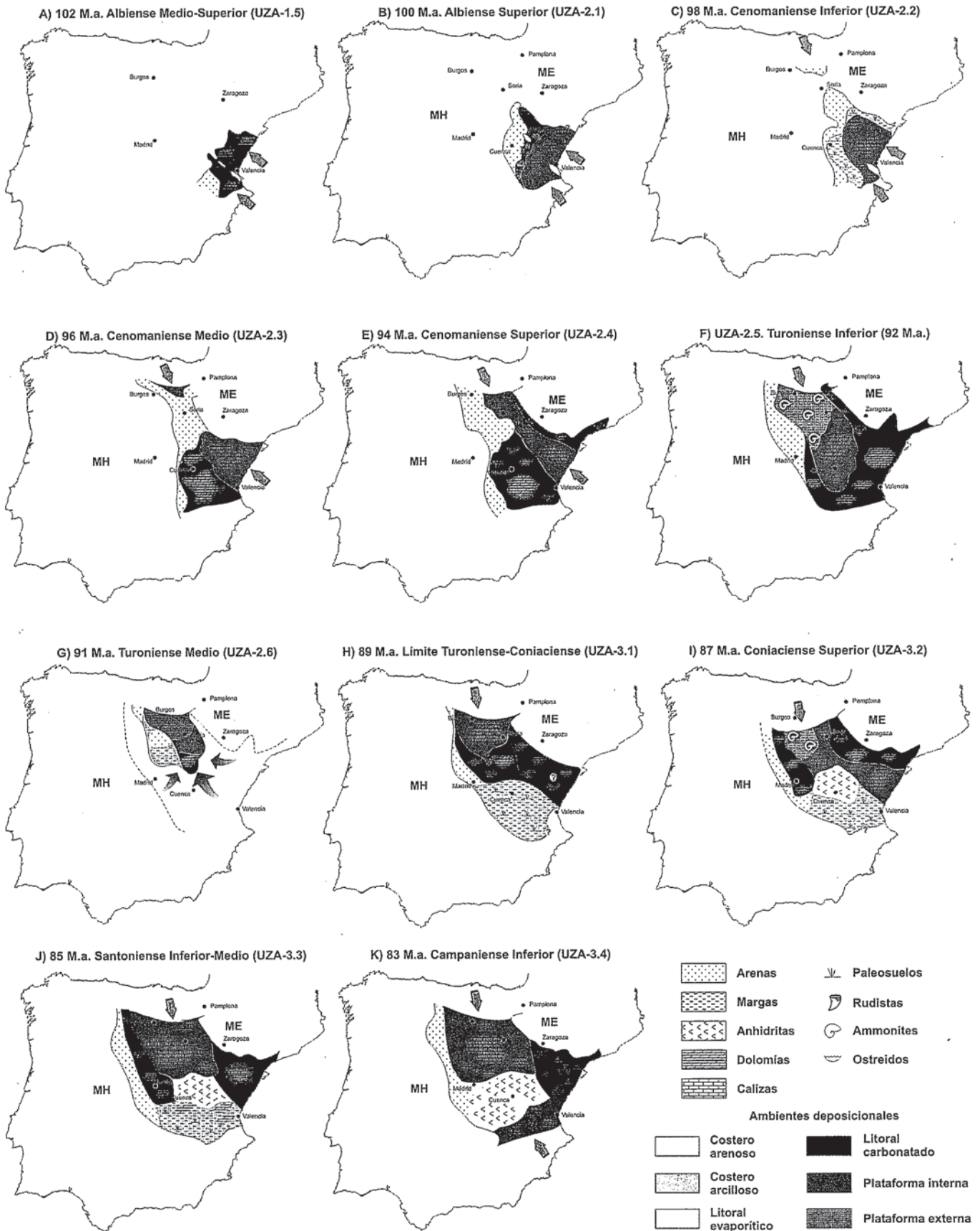
Fig. 2.- Mapas paleogeográficos y distribución de facies de la Cuenca Ibérica de los once episodios deposicionales de 3 er orden diferenciados entre el Albiense superior- Campaniense inferior.
