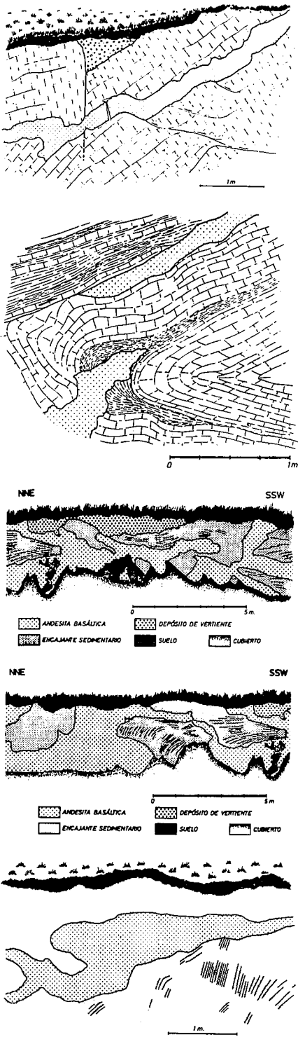
Fig. 2.—Modalidades del emplazamiento de intrusiones: a) originando desplazamientos en el sedimento encajante, b) afectando a pliegues, c) con desarrollo digitado, d) englobando al sedimento encajante y e) con estructuras de acomodación.
