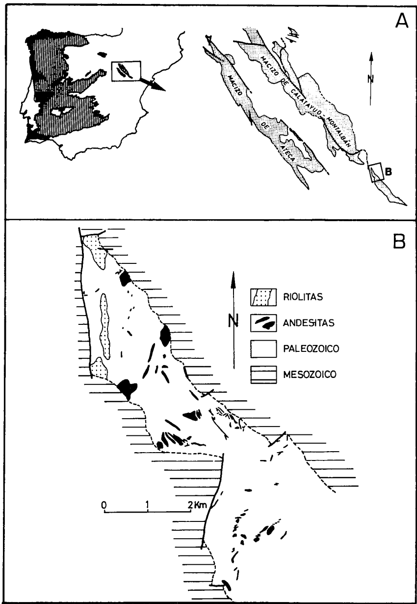
Fig. 1.—Localización geológica del área: A) Unidad de Montalbán, B) Cartografía de las intrusiones en el Sector N del Anticlinal de Montalbán.
