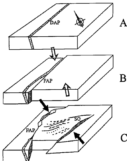
Fig. 3.- Modelo de evolución de la falla Alentejo-Plasencia en Extremadura, antes del Terciario (A), durante el Paleógeno (B) y durante el Aragoniense medio (C). Flechas, dirección de compresión. FAP, Falla de Alentejo-Plasencia. DAP, dique de Alentejo-Plasencia. SG, bloque de la Sierra de Guadalupe.
