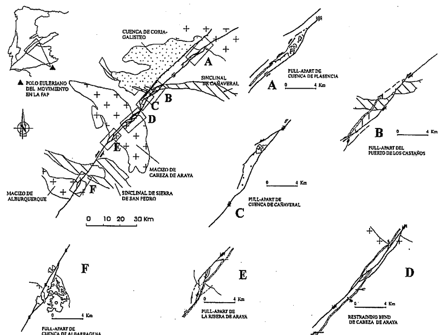
Fig. 1.- Situación en el macizo Hespérico, geometría general y estructuras asociadas a inflexiones de la Falla de Alentejo-Plasencia. A, pull-apart de Plasencia. B, pull-apart del Puerto de los Castaños. C, Pull-apart de Cañaverall. D, Restraining bend of Cabeza de Araya. E, Pull-apart de Ribera de Araya. F, Pull-apart de Albarragena.
