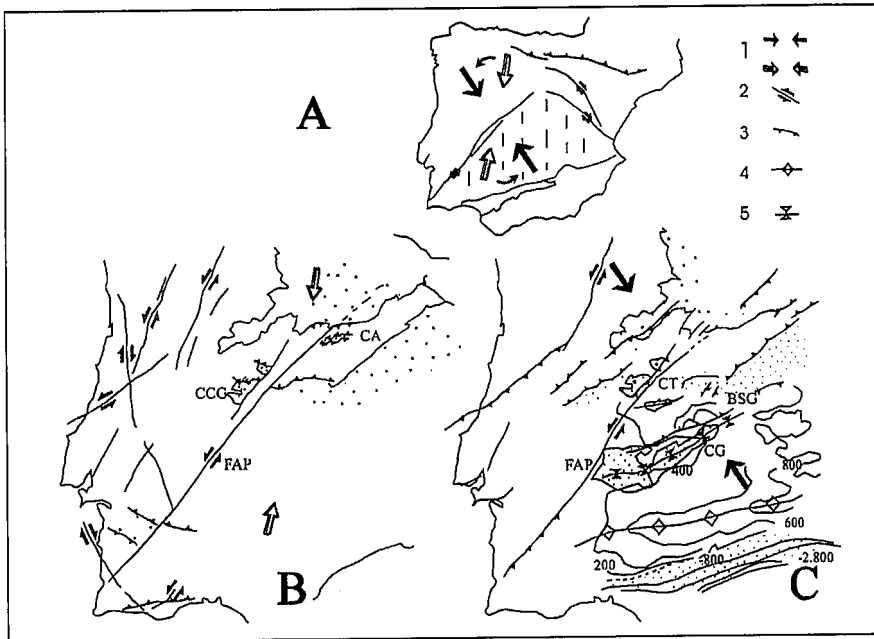
Fig. 2.- Evolución de la Falla de Alentejo-Plasencia durante las dos etapas principales de compresión alpina. A, Situación general, con el bloque central de la Meseta limitado por desgarres laterales, uno de ellos la FAP. B, Fallas inversas y desgarres activos durante la compresión paleógena. La FAP muestra traza rectilínea. C, Fallas activas durante la compresión miocena (Aragoniense medio). La FAP se incurva y se forman las cuencas pull-apart. Se levanta también el bloque de la Sierra de Guadalupe (BSG). C.C.G., cuenca de Coria-Galisteo. C.A., Cuenca del Amblés. C.T., Cuenca de Talaván. B.S.G., Bloque de la Sierra de Guadalupe. 1, direcciones de compresión. 2, desgarre. 3, falla inversa. 4, elevación tectónica. 5, depresión.
