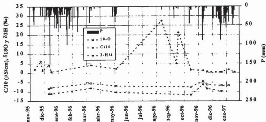
Fig. 3.- Evolución temporal de la conductividad eléctrica y de los contenidos en ^{18}\text{O} y ^2\text{H} del agua de lluvia muestreada en la estación de Cuevas del Moro.
