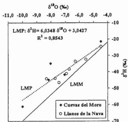
Fig. 2.- Diagrama \delta^2\text{H} y \delta^{18}\text{O} de las muestras de precipitación. (LMM) línea meteórica mundial, (LMP) línea meteórica local.
